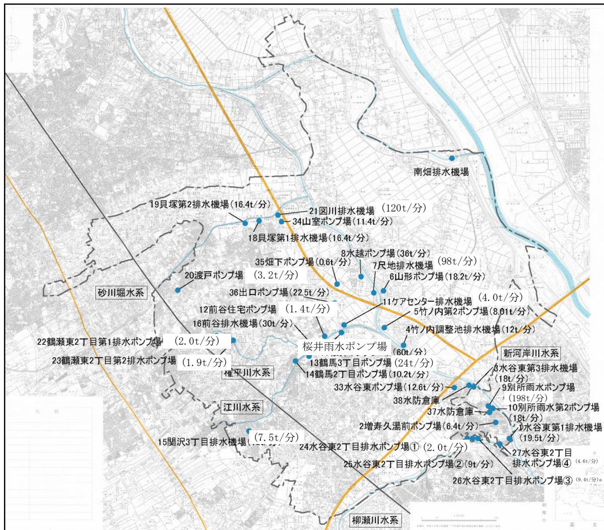
資料67 水防施設配置図
