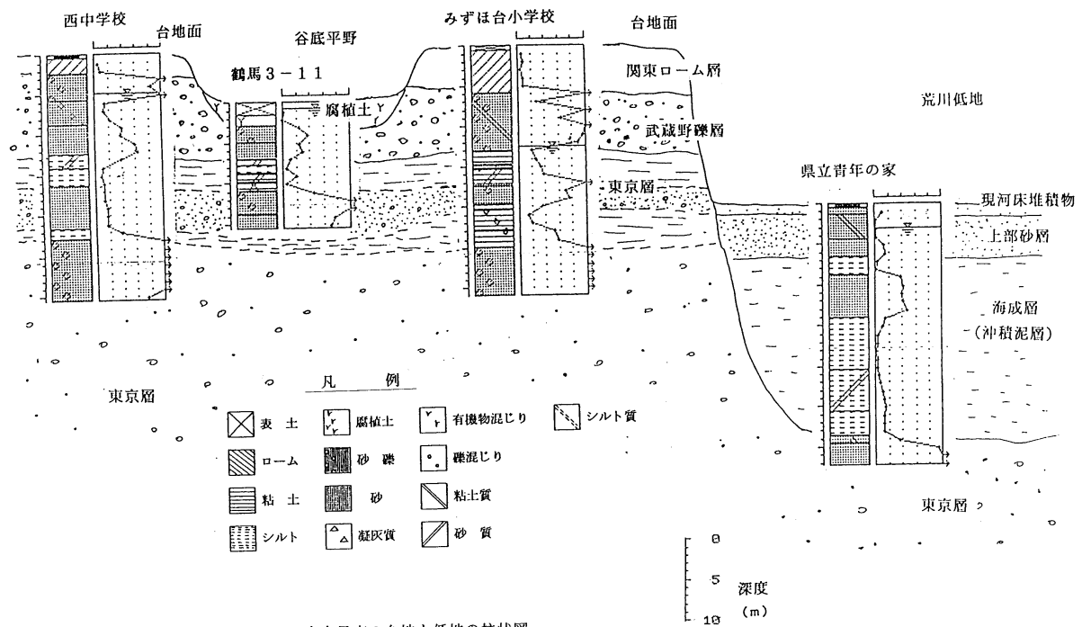
図1-1 富士見市の台地と低地の柱状図 (平成2年度 防災アセスメント調査による)
